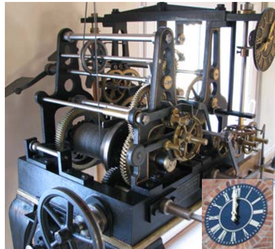
Zweivalzenwerk mit elektrischem Aufzug und einer funktechnischen Steuerung
